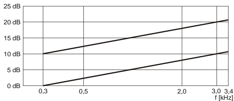
Rys.8. Charakterystyka częstotliwościowa toru nadawczego
