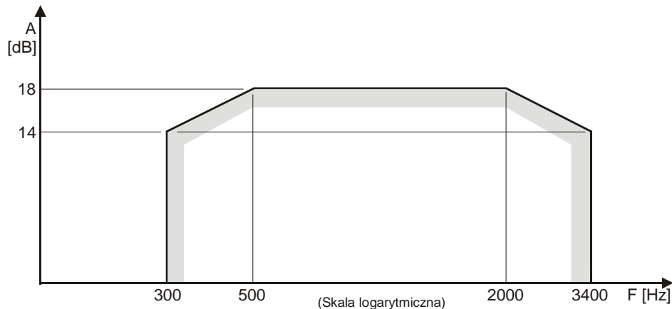
Rys. 3. Minimalna wartość tłumienności niedopasowania
