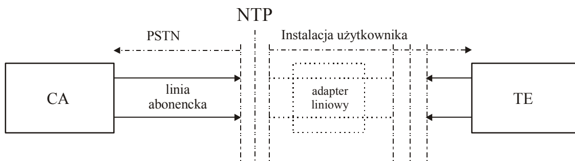
Rys.1 Punkt dostępu do sieci PSTN
