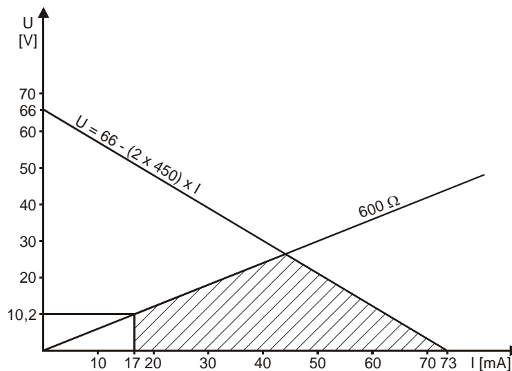
Rys. 2. Wartość dopuszczalnej rezystancji urządzenia końcowego
